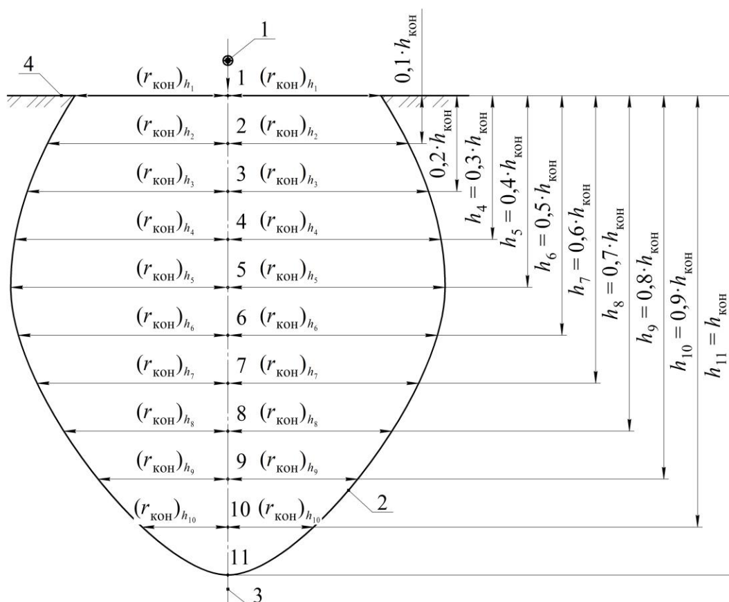
1 – капельница; 2 – оконтуривающая линия; 3 – ось капания; 4 – поверхность земли; h_1 - h_{11} – расстояния от поверхности земли до разделяющих контур сечений, м; (r_{\text{кон}})_{h_1} - (r_{\text{кон}})_{h_{11}} – соответствующие сечениям радиусы контура, м; 1 – 11 – точки на оси капания, соответствующие сечениям контура
