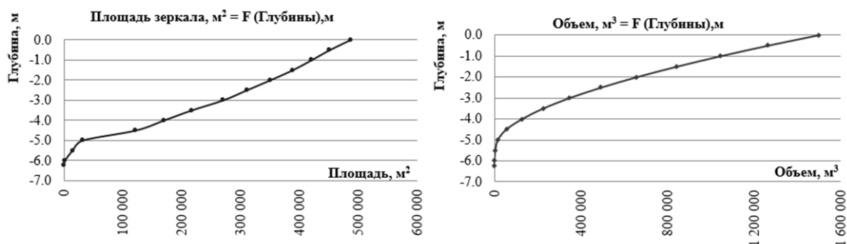
Рисунок 2 – Батиграфические зависимости
