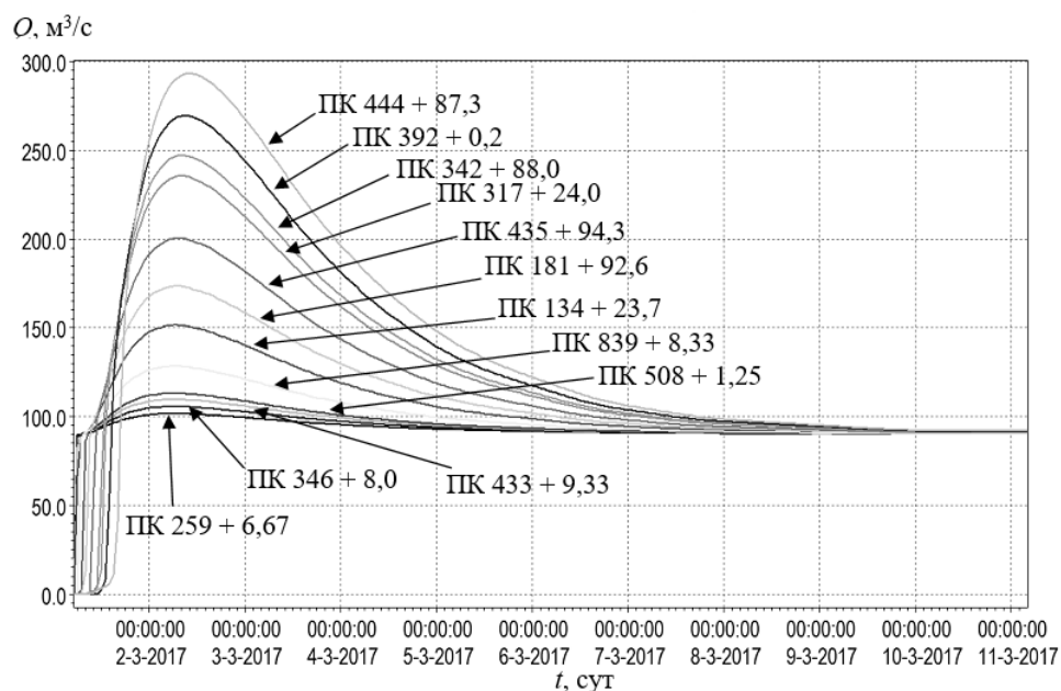
Рисунок 3 – Графики прохождения максимальных расходов при 3,0 % обеспеченности стока
