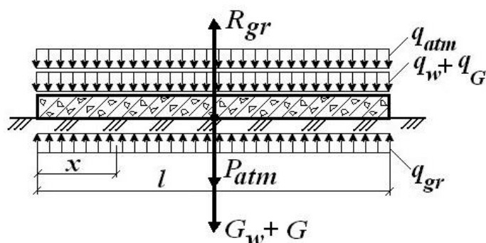
Рисунок 3 – Схема силового воздействия на плиту крепления дна
