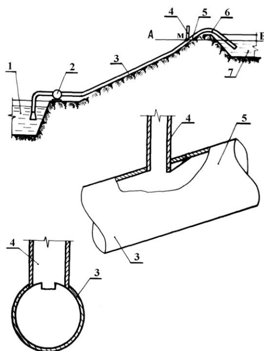
Рисунок 1 – Схема установки аэрационной трубы
