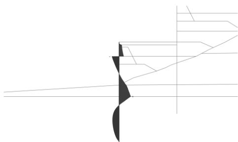
Рисунок 12 – Эпюра поперечных усилий в лицевой стенке
