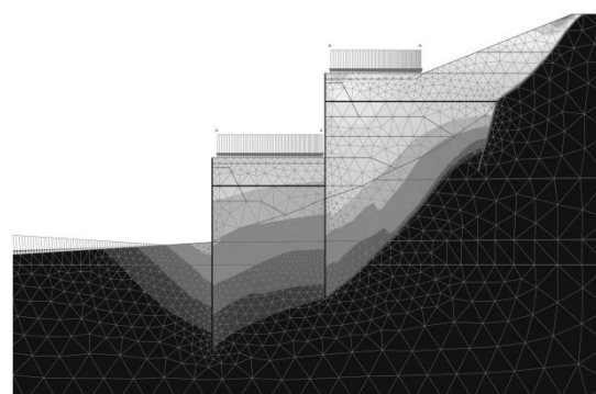
Рисунок 7 – Форма прогнозируемого обрушения
