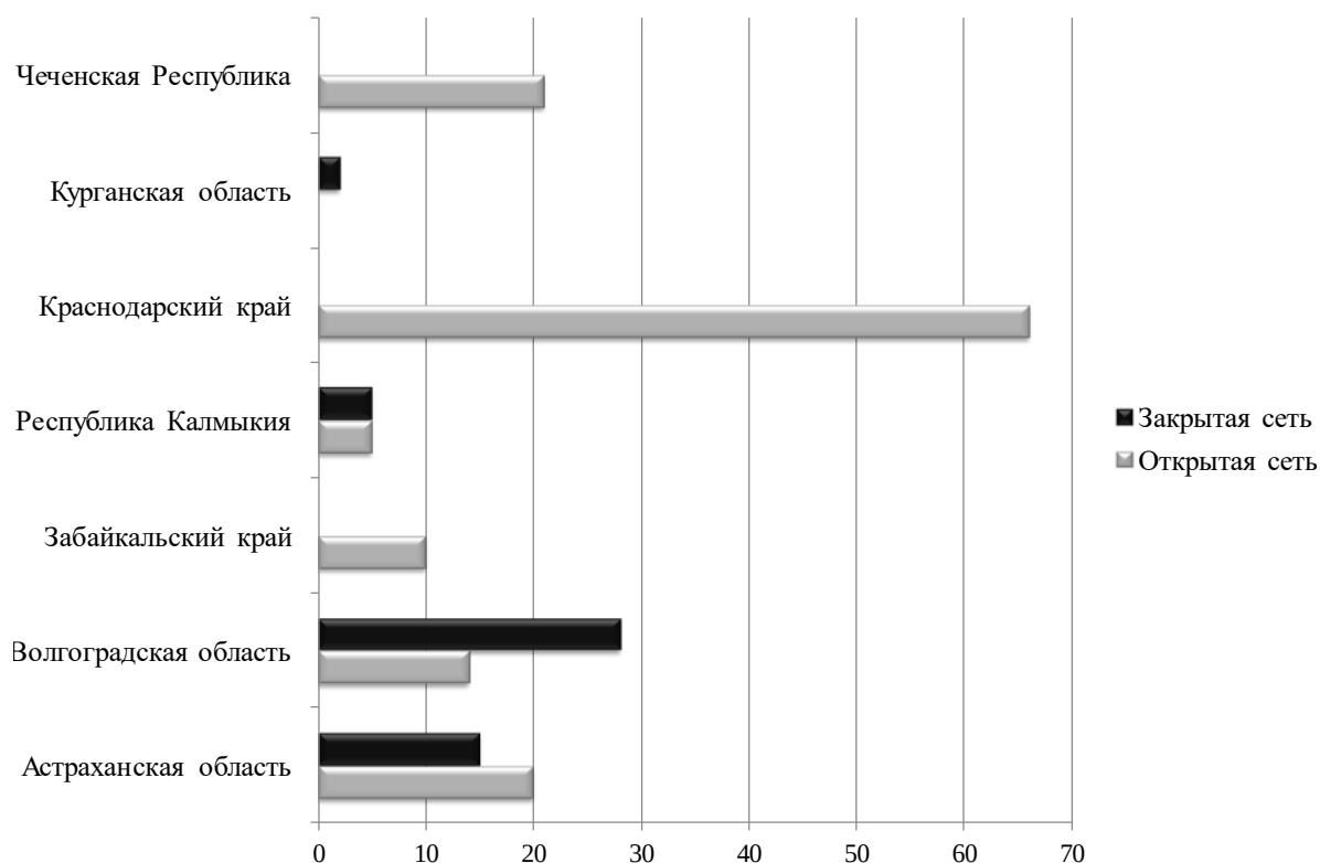
Рисунок 4 – Потребность в строительстве пунктов водоучета на мелиоративных системах Минсельхоза России по субъектам Российской Федерации и условиям применения
