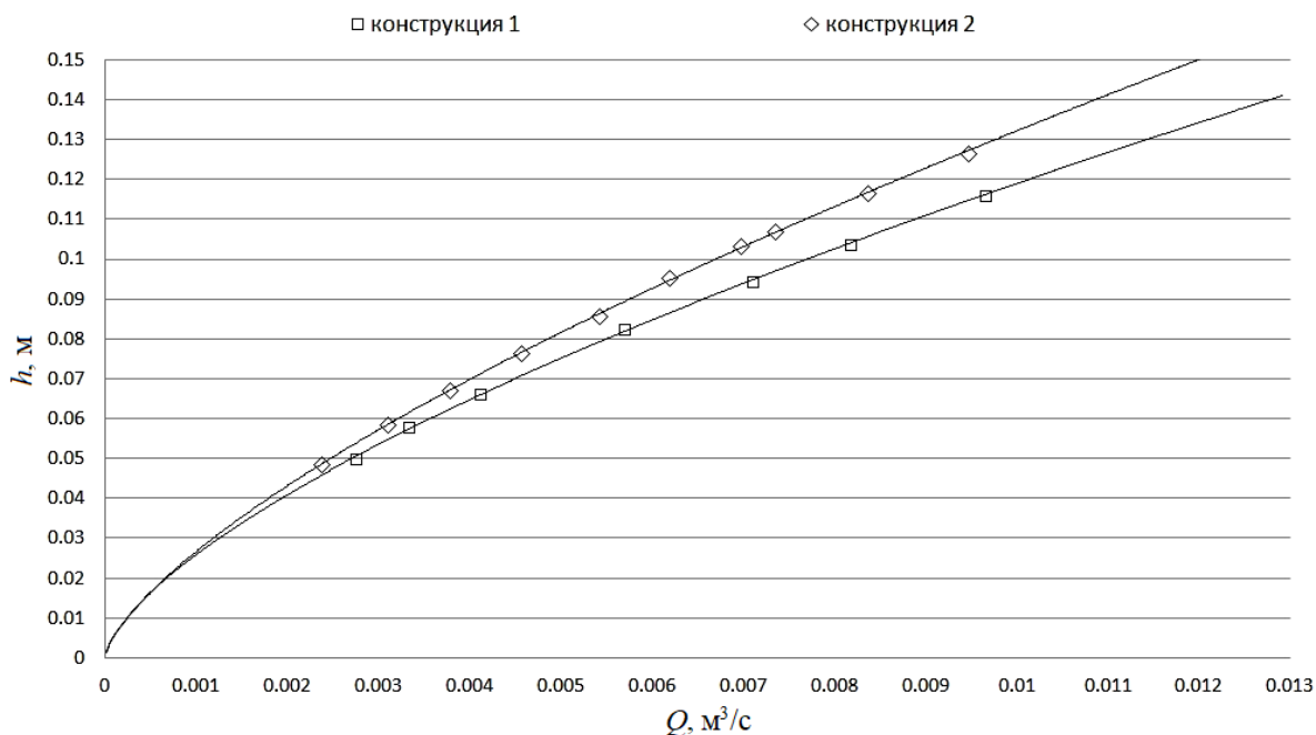
Рисунок 2 – Кривые зависимости напора от расхода
