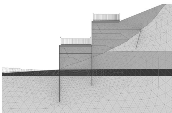
Рисунок 6 – Расчетная схема
