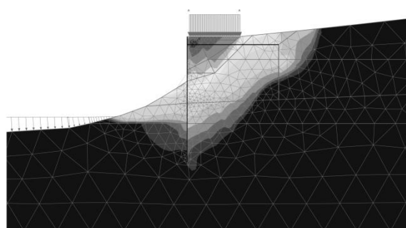
Рисунок 2 – Форма прогнозируемого обрушения
