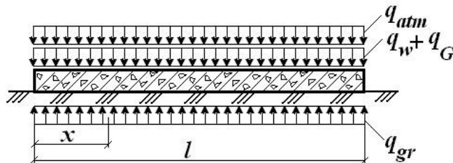
Рисунок 1 – Схема нагрузок, действующих на плиту в поперечном направлении
