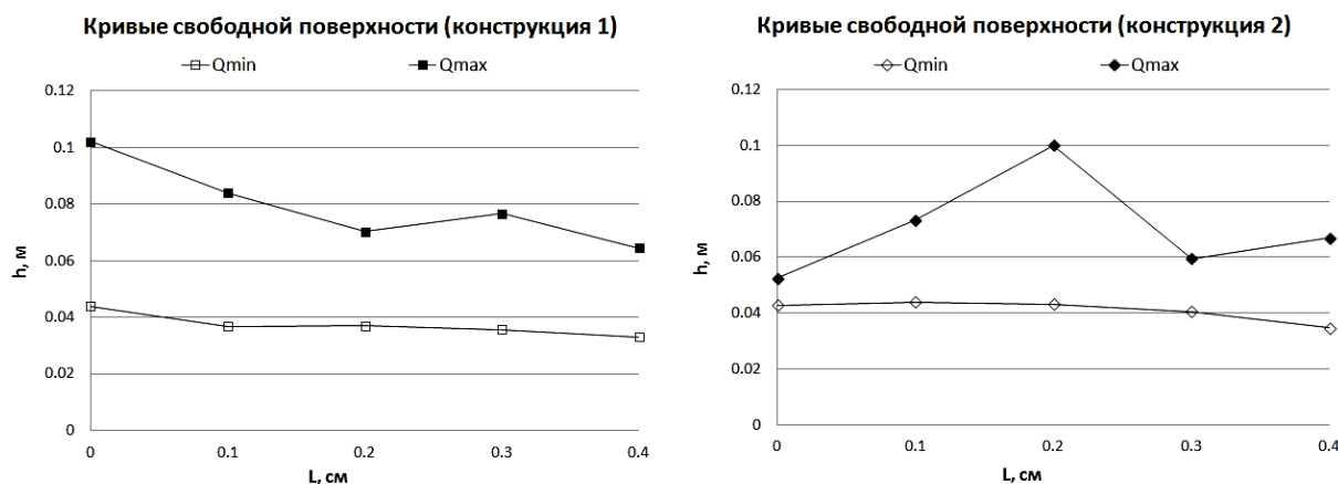
Рисунок 3 – Кривые свободной поверхности в горловине
