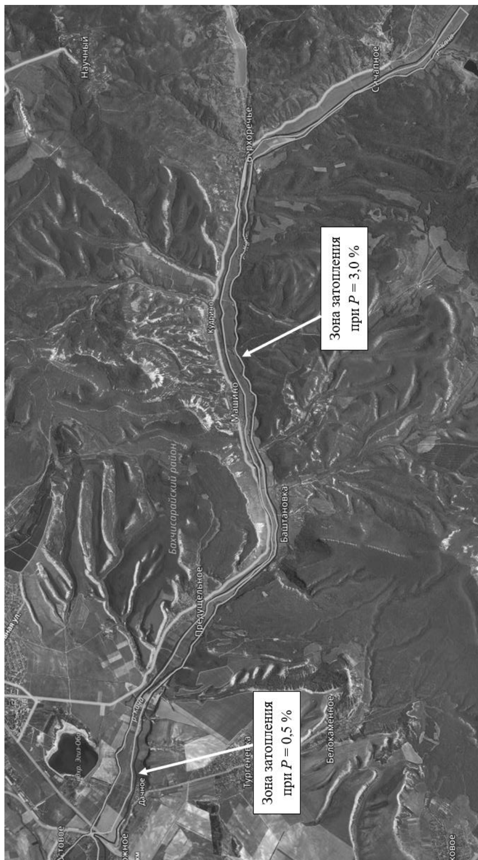
Рисунок 4 – Зоны затопления на рассматриваемом участке р. Качи (ПК 0 – ПК 19670)
