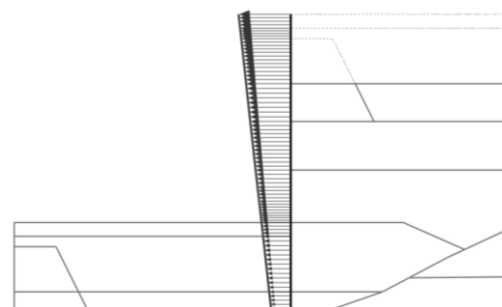
Рисунок 7 – Форма прогнозируемого обрушения
