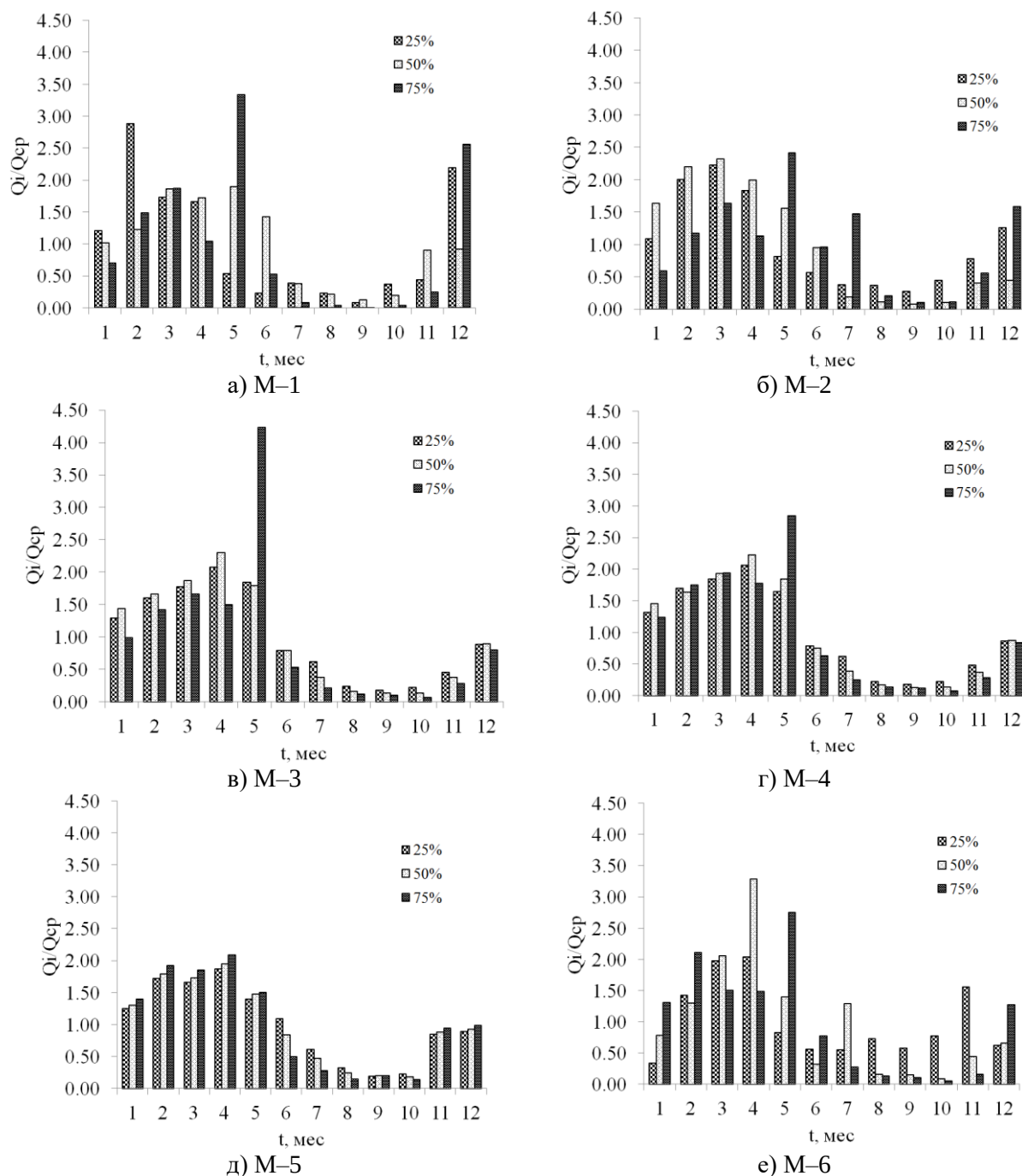
Рисунок 1 – Графики внутригодового распределения (гидрографы) стока при использовании различных расчетных методов при обеспеченности стока 25, 50, 75 %
