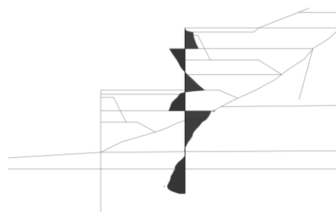
Рисунок 13 – Эпюра поперечных усилий в верхней стенке
