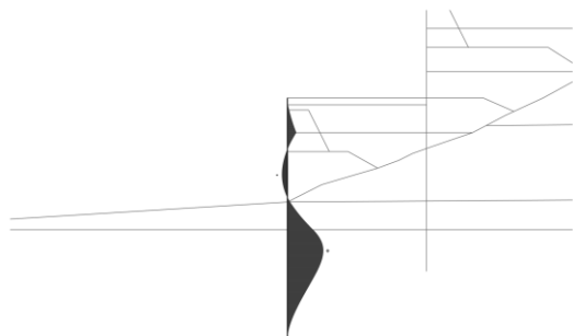
Рисунок 8 – Полные горизонтальные смещения в лицевой стенке
