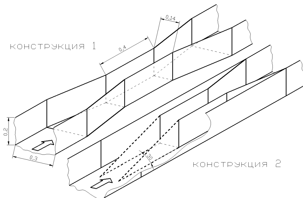
Рисунок 1 – Конструкции 1 и 2 входной части лотка критической глубины
