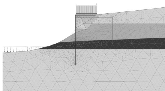
Рисунок 1 – Расчетная схема
